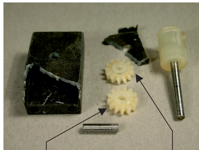
Zahnrad mit grösserem Innendurchmesser
