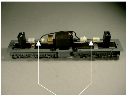
Kardanwellen müssen ca. 0.5 mm Längsspiel aufweisen
