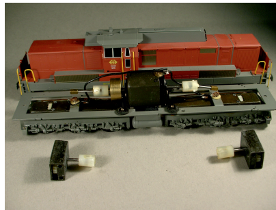
Fulgurex Am6/6 mit ausgebauten Original Getrieben
