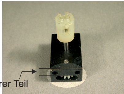
Randrierung muss im dickeren Teil des Getriebes sein
