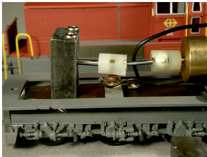
verbogenes Getriebe
